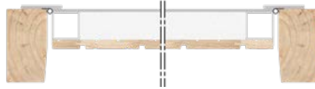
Horizontalsnitt vipport med alu-stomme
